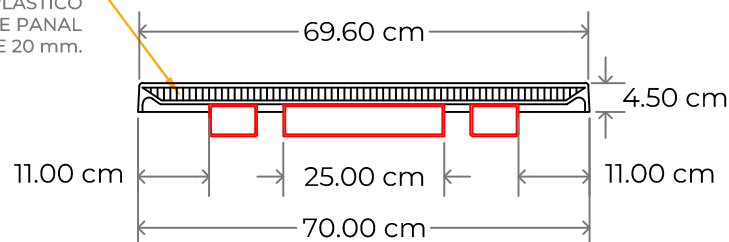
CORTE FRONTAL TAPA
