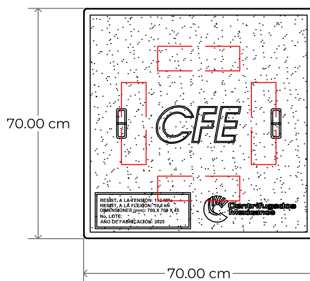
VISTA SUPERIOR TAPA
