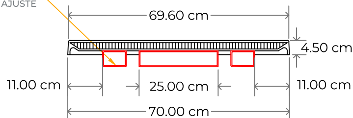
CORTE LATERAL TAPA
