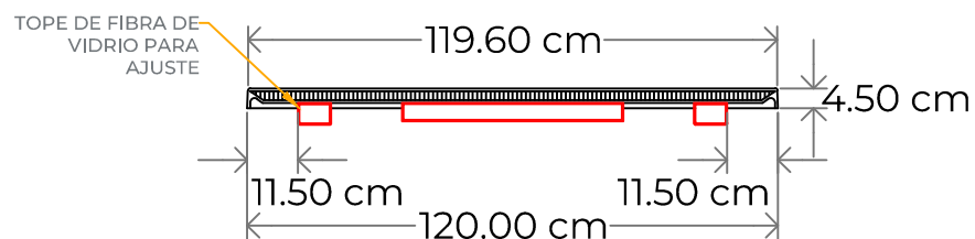
CORTE LATERAL TAPA
