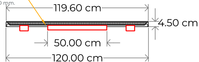
CORTE FRONTAL TAPA
