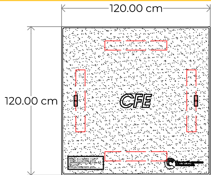
VISTA SUPERIOR TAPA
