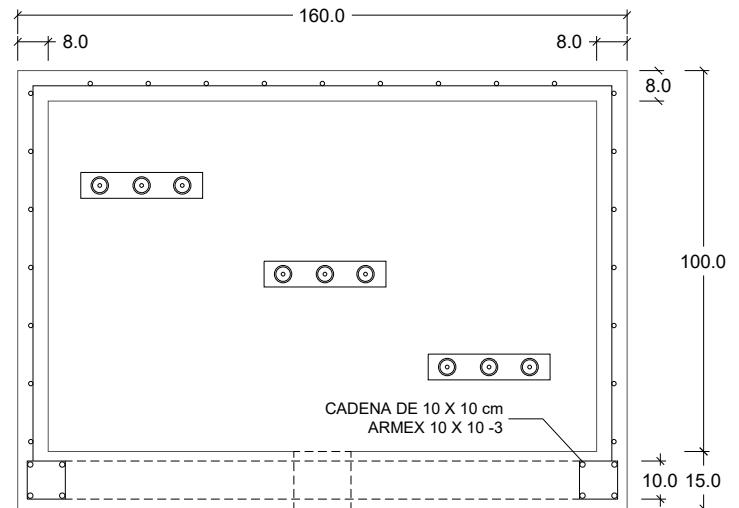
Detalle Frontal
