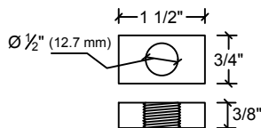
Detalle Tuerca
