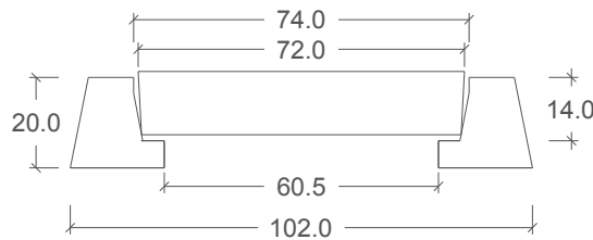
Detalle Ensamble
