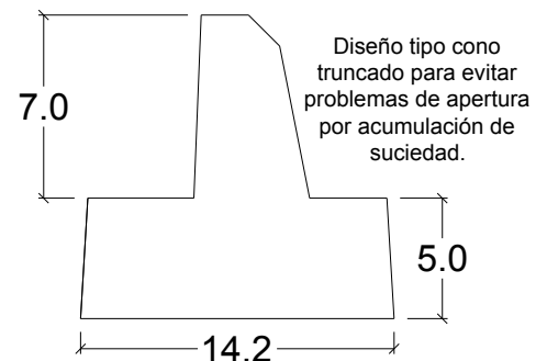
Detalle Marco
