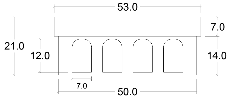
Vista Lateral Registro
