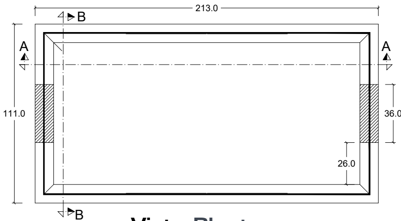
Vista Planta
