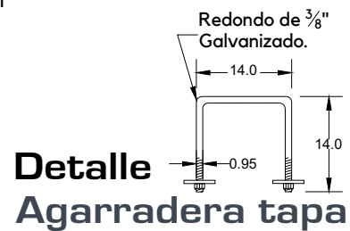
Alzado Tapa
