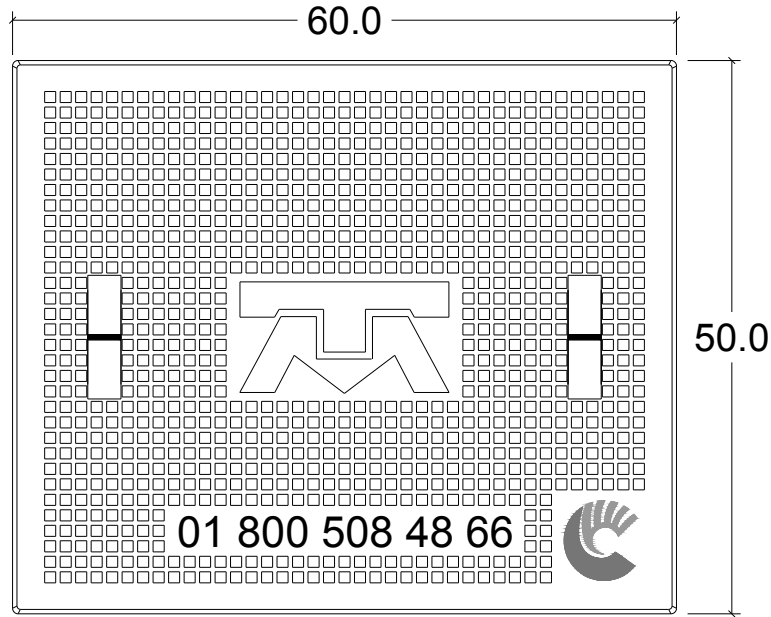
Vista Planta Tapa
