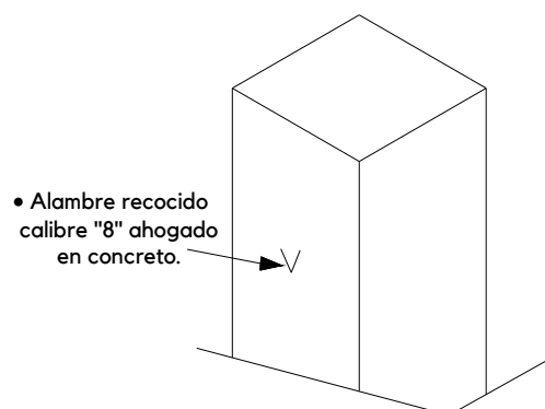
Detalle 1
