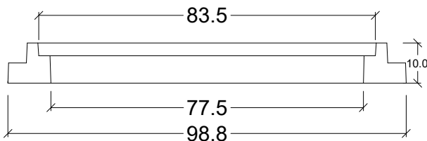
Vista Lateral Aro
