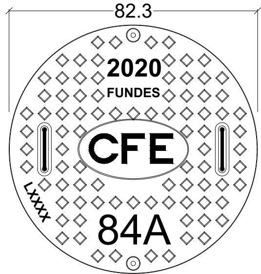
Vista Planta Tapa
