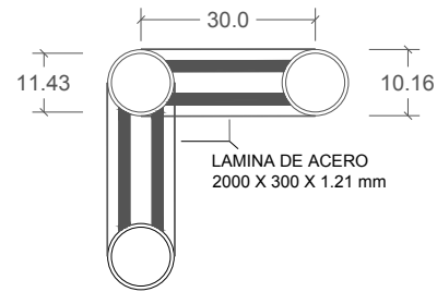
Detalle Armado de torre con 3 apoyos
