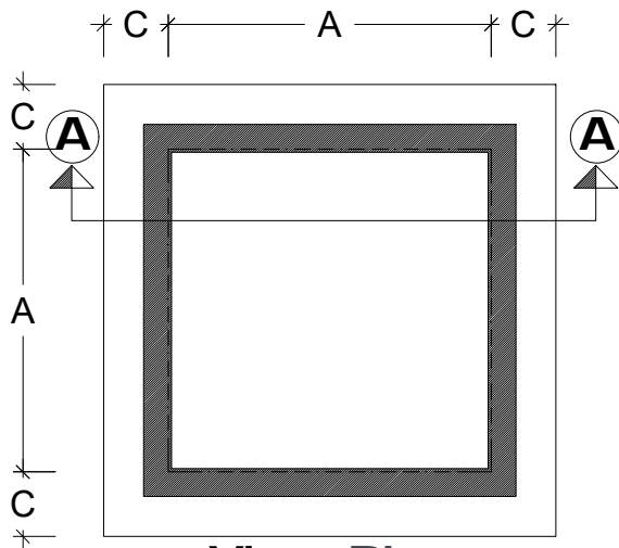
Vista Planta
