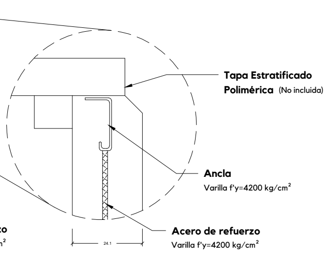
Detalle 1
