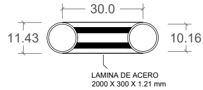
Detalle Armado de torre con 3 apoyos
