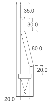
Detalle Punta
