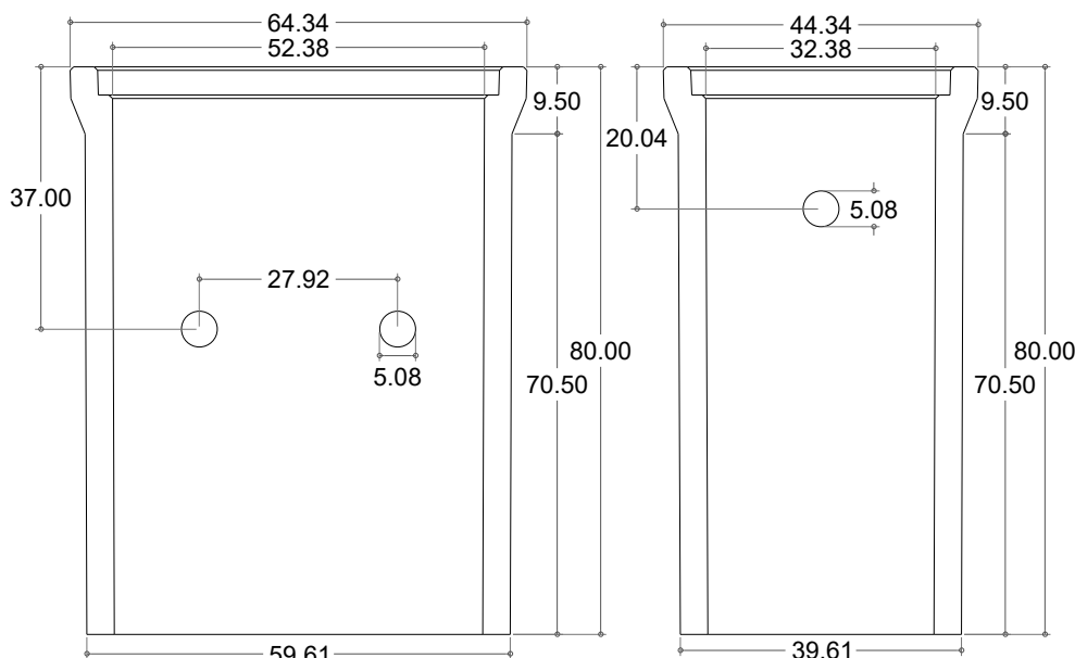
Corte A-A'
