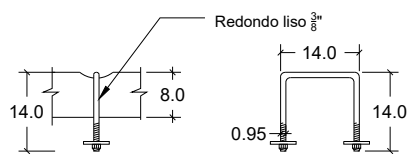
Detalle Agarraderas
