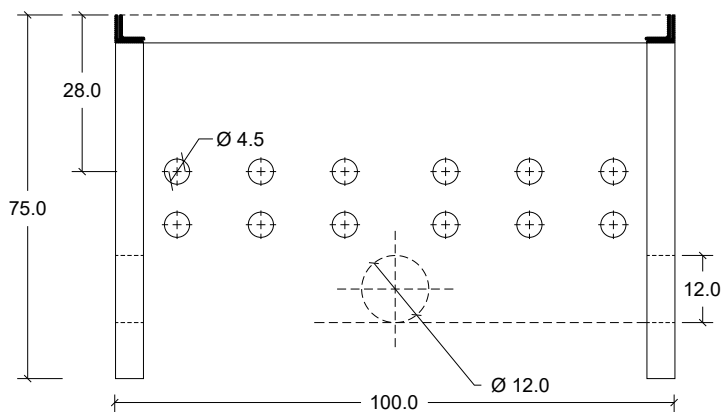
Corte B-B
