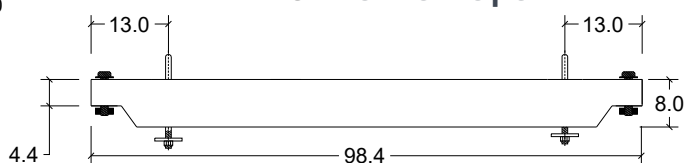
Alzado Tapa
