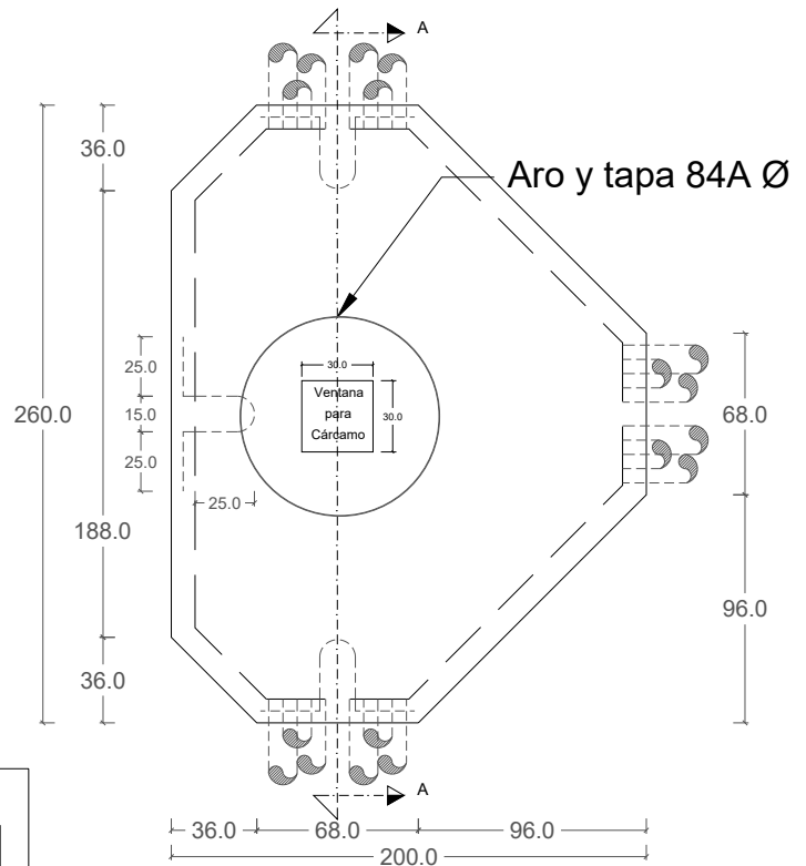
Vista Planta
